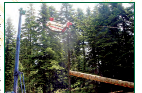
Débardage d'une grume par câble
